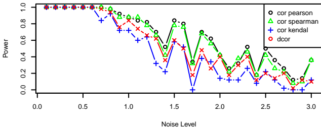
Cubic
